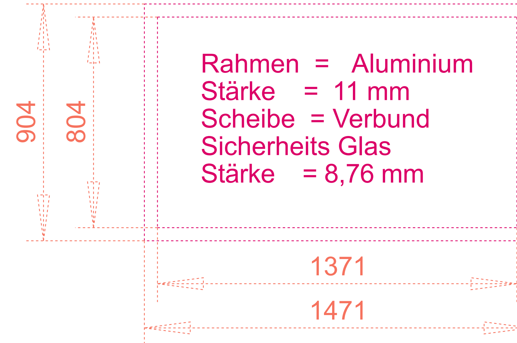
Glas Kasette kurze Seite
