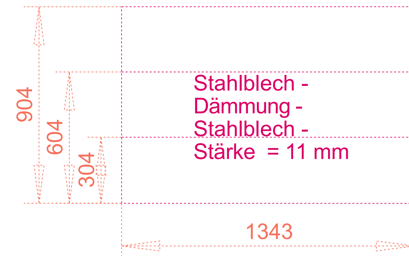
Standard Kasette kurze Seite
