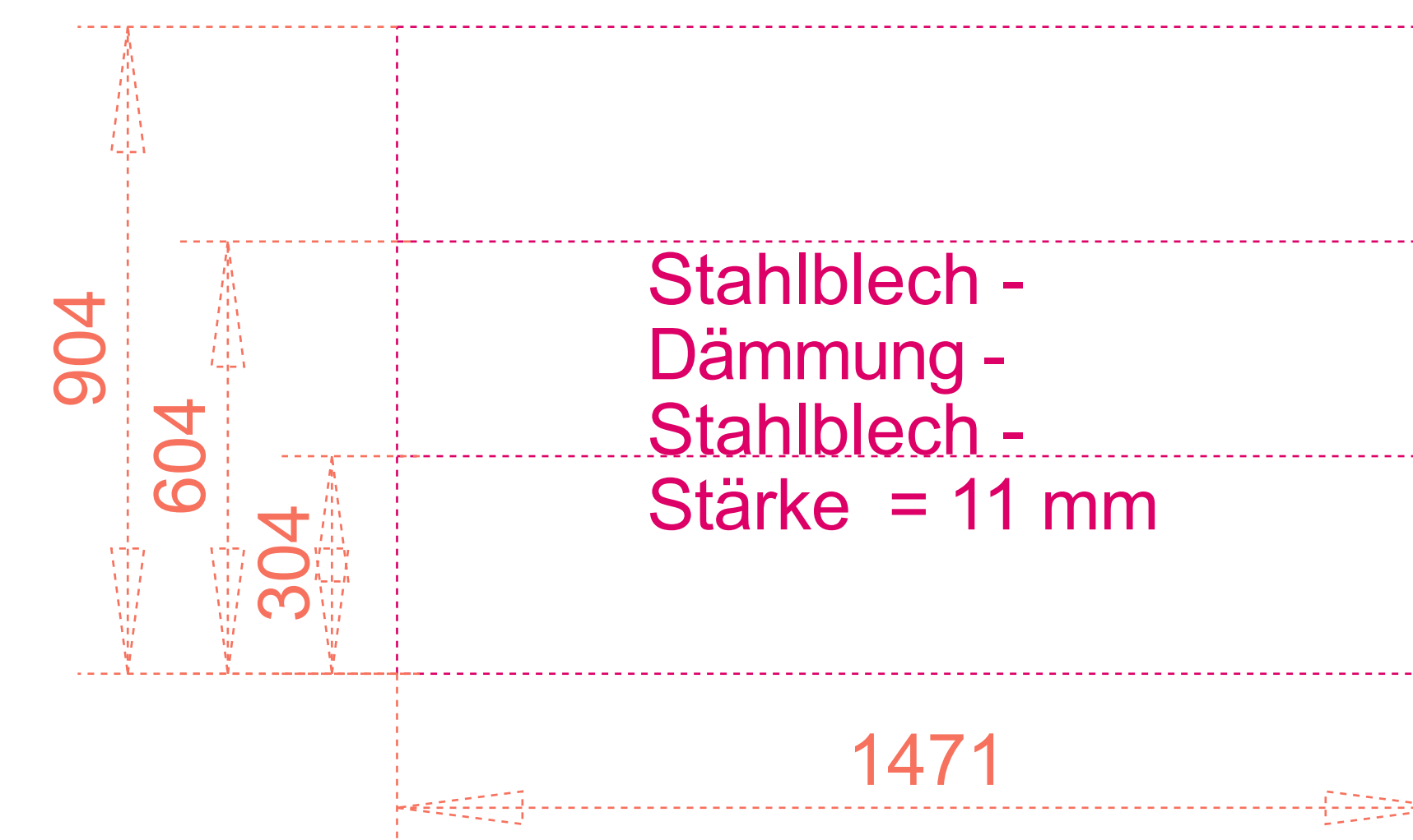
Standard Kasette lange Seite
